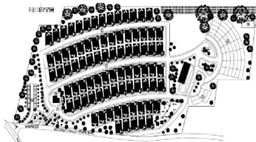
Figura 28. Iztapa, Plano de Conjunto
