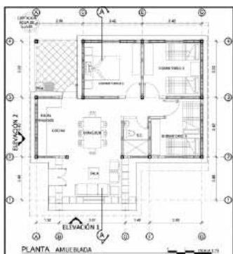
Figura 29. San Marcos, Planta de la Propuesta
