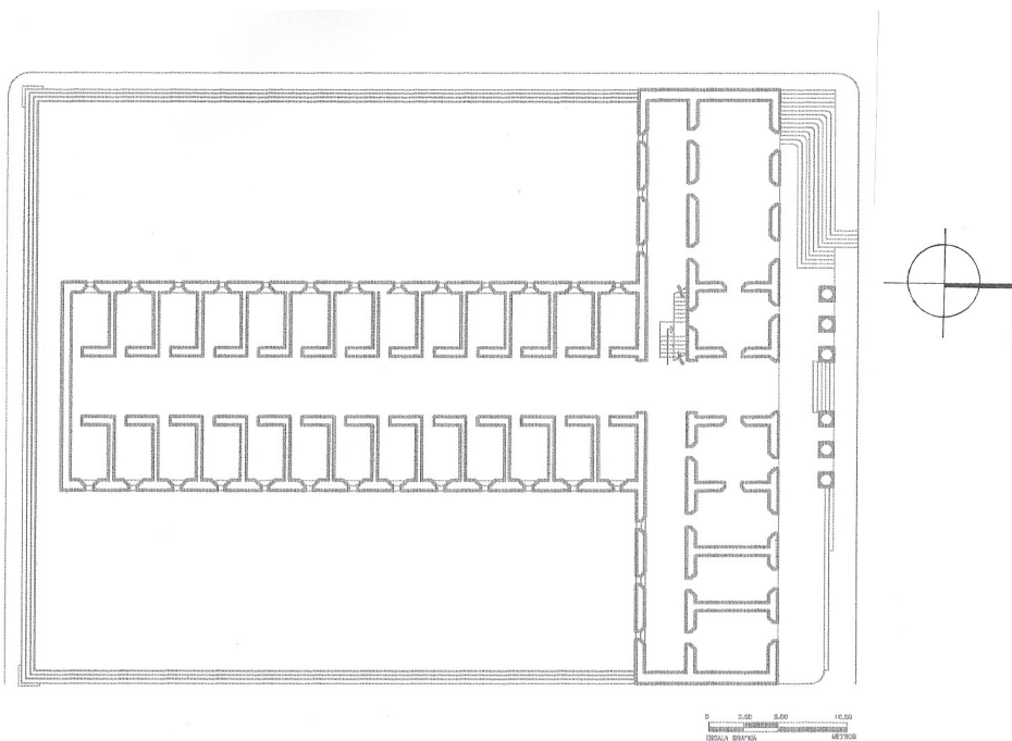
Imagen 02. Planimetría de Omar Maldonado Valle. Planta baja de la Penitenciaría de Occidente. Obsérvese la estrechez de los espacios interiores con entresijos de madera a diferencia de la monumentalidad de la fachada principal. 1998. Tomada del trabajo de tesis de la Facultad de Arquitectura de la USAC.
