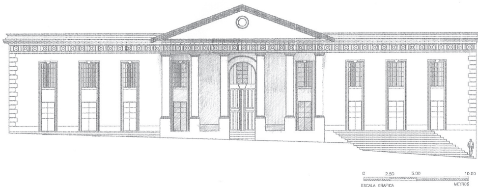
Imagen 01. Planimetría realizada por Omar Maldonado Valle con sombreados del autor. Fachada principal de la antigua Penitenciaría de Occidente al sur de la plaza mayor de Quetzaltenango. 1998. Tomada de la tesis de grado de arquitecto de la USAC.
