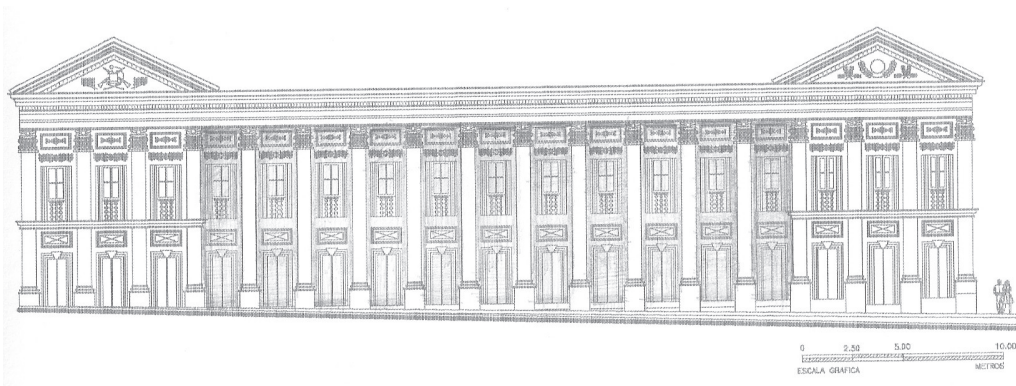
Imagen 03. Planimetría de Omar Maldonado Valle con sombreados de Carlos Ayala R. Alzado frontal del Palacio municipal de Quetzaltenango. 1998. Tomado de la tesis de grado de la Facultad de Arquitectura de la USAC.
