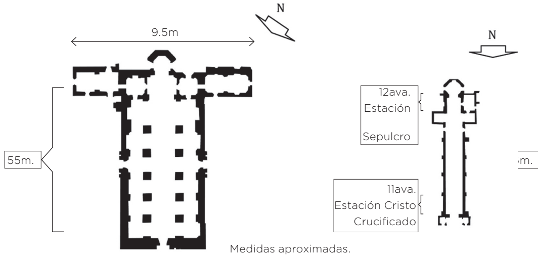
Figura 4 Esquema de la planta arquitectónica del templo del Calvario, La Antigua Guatemala.
